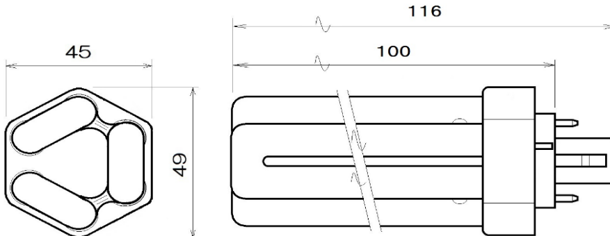
図-1 (単位:mm)
