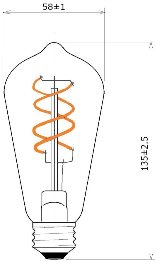
図-1 (単位:mm)
