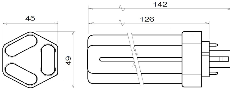
図-1 (単位:mm)
