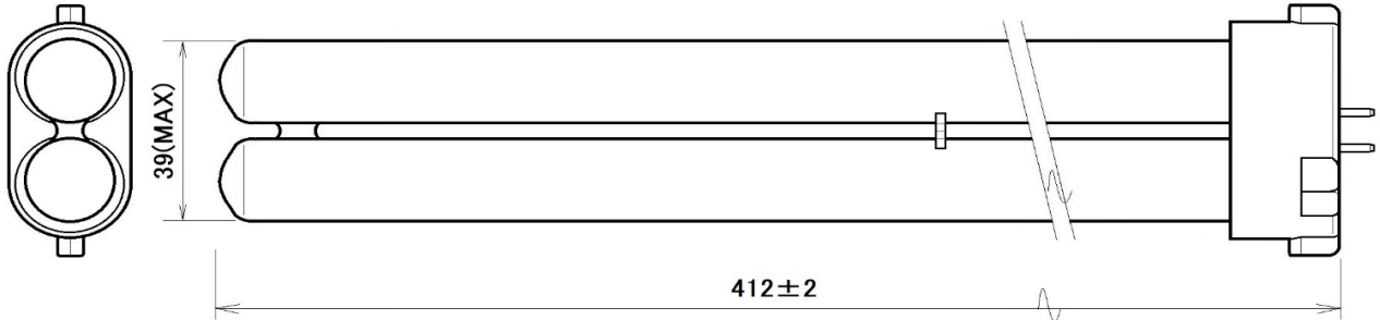
図-1 (単位:mm)
