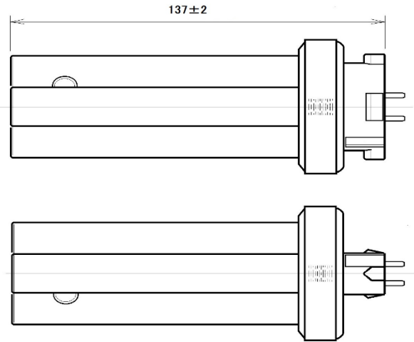
図-1 (単位:mm)
