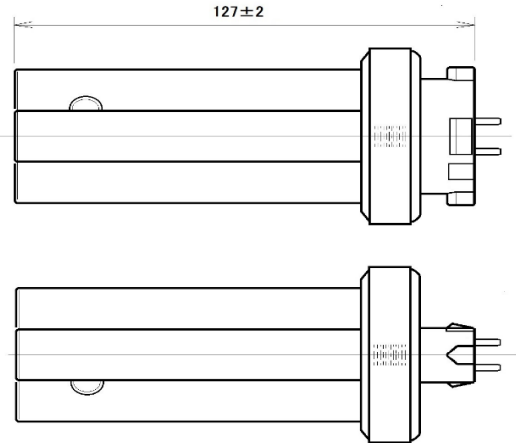
図-1 (単位:mm)
