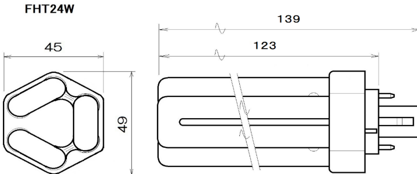
図-1 (単位:mm)
