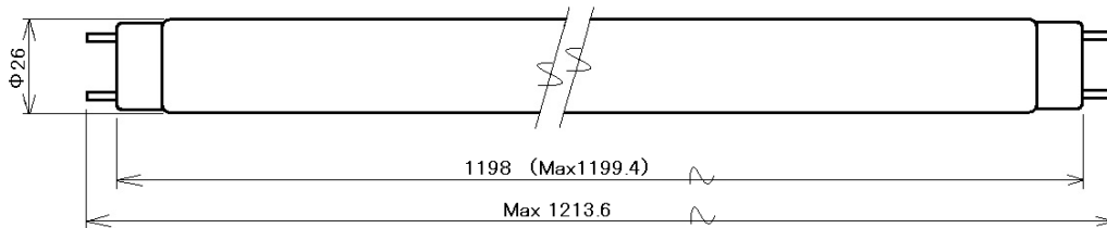
図-1 (単位:mm)
