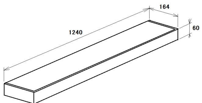
図-2 (単位:mm)
