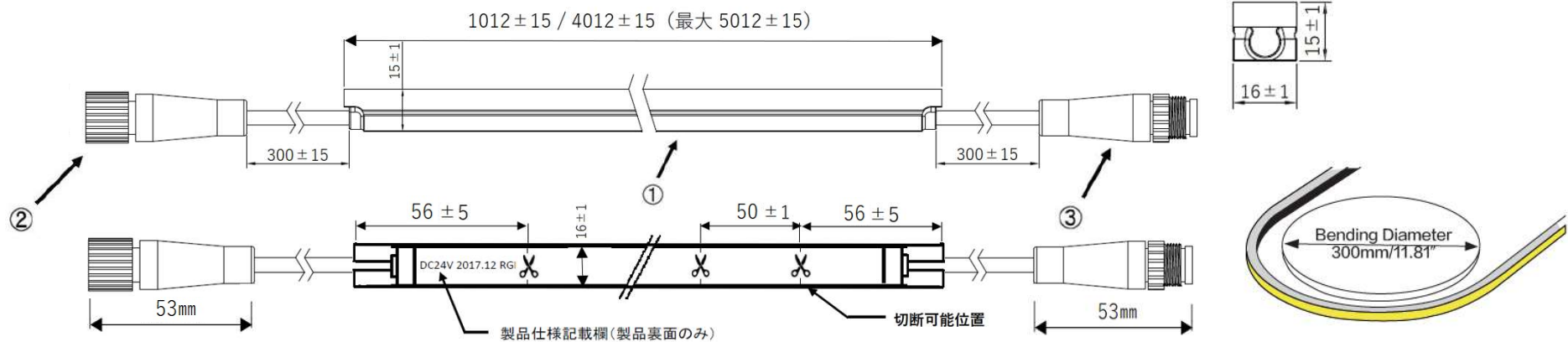
付属品部品
