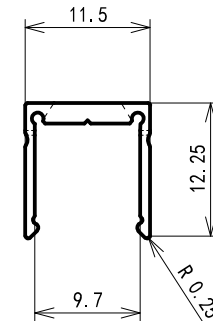
右视图1
